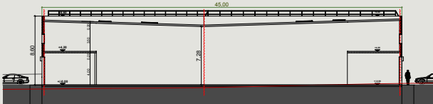
Coupe C2C2
