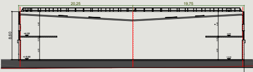
Coupe C3C3
