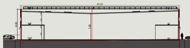
Coupe C2C2
