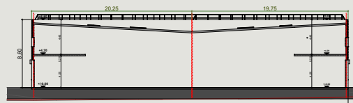
Coupe C3C3
