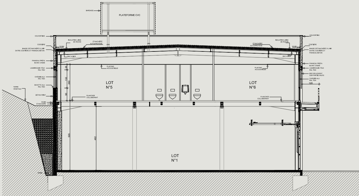
COUPE BB
