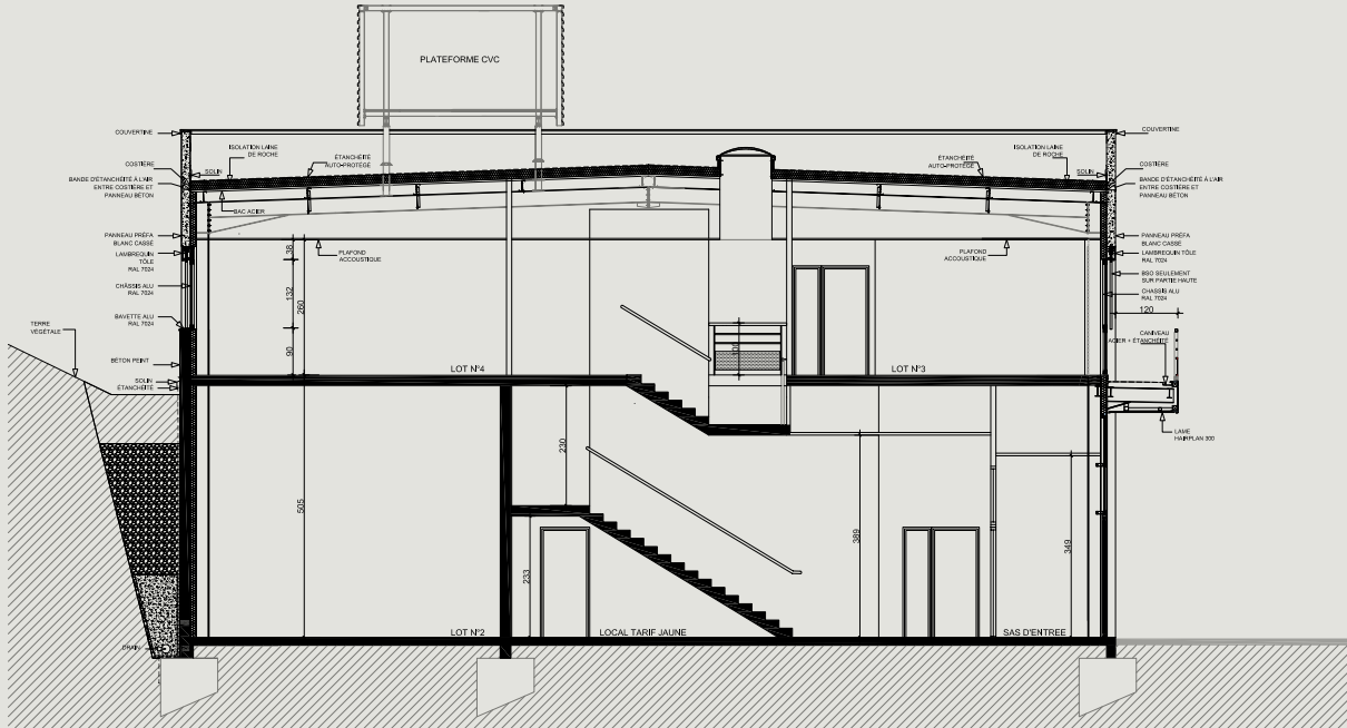
COUPE AA
