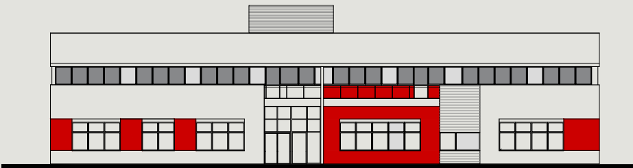
FAÇADE OUEST
