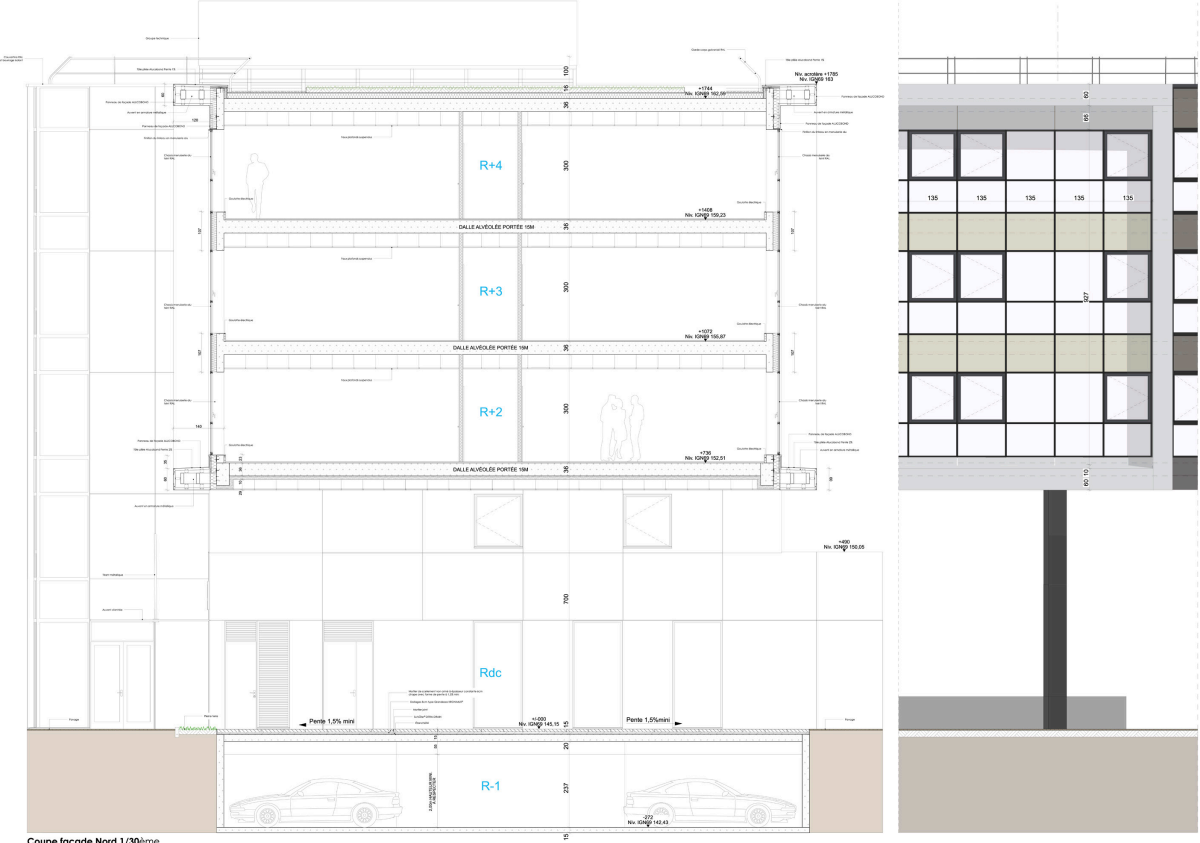
Coupe façade Nord 1/30ème
